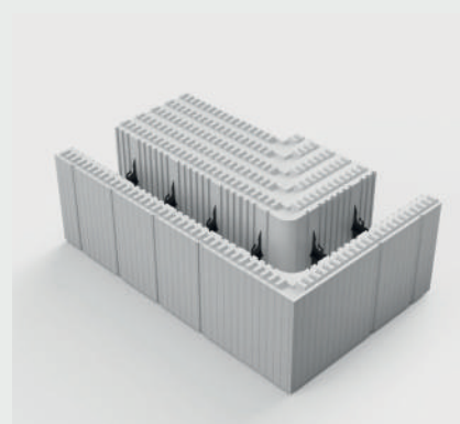
BLOC ANGLE RENTRANT 90°
