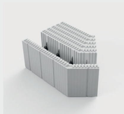
BLOC ANGLE RENTRANT 45°
